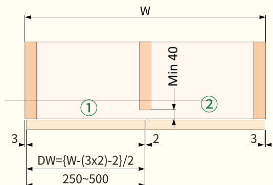
Door Widths
